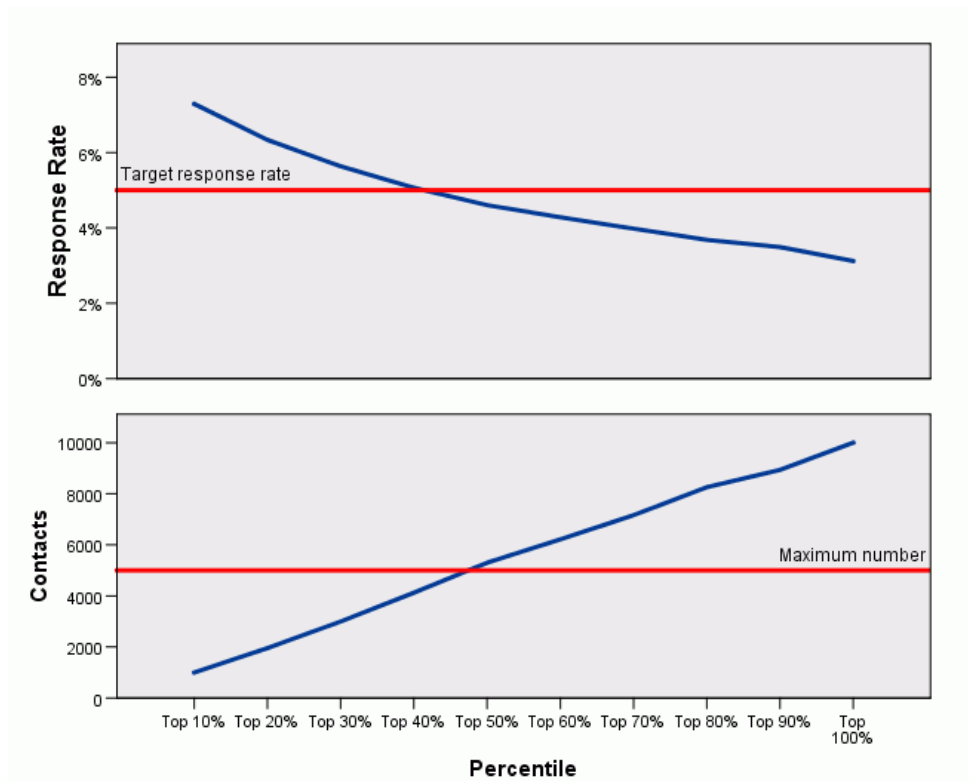
图片 11-6 累积响应率图表
