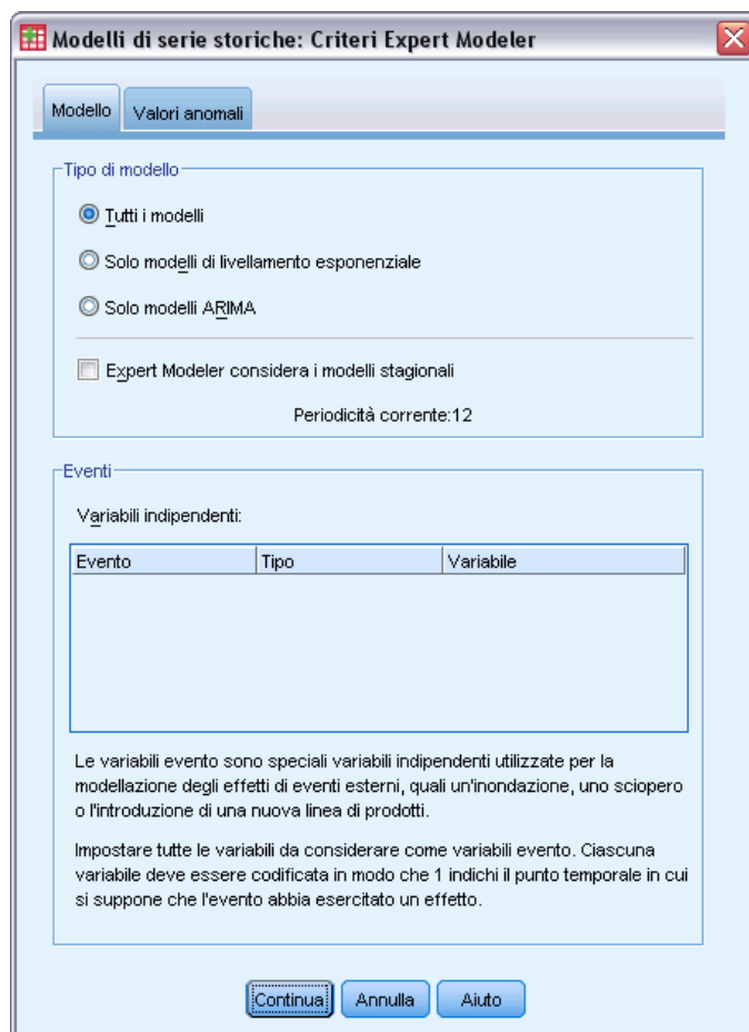
Figura 2-2 Finestra di dialogo Criteri di Expert Modeler, scheda Modello
