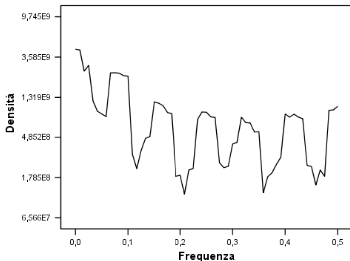
Figura 11-4 Densità spettrale
