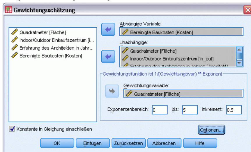
Abbildung 6-1 Dialogfeld "Gewichtungsschätzung"
