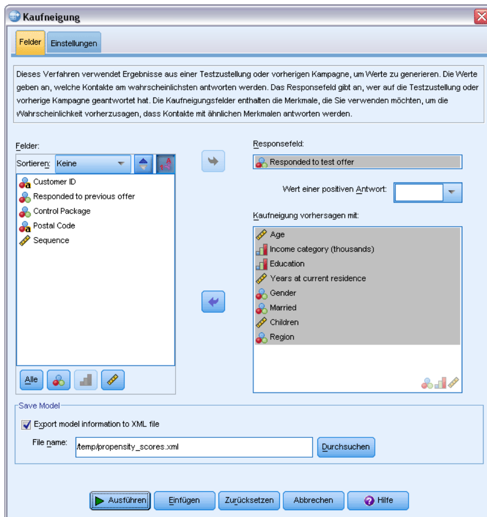
Abbildung 6-3 Kaufneigung, Registerkarte "Felder"
