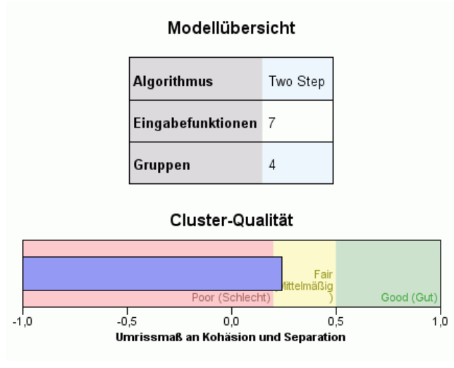
Abbildung 9-3 Cluster-Modellzusammenfassung
