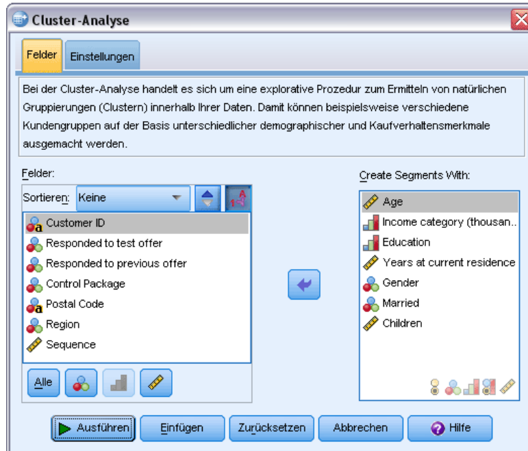
Abbildung 3-2 Registerkarte "Clusteranalysefelder"
